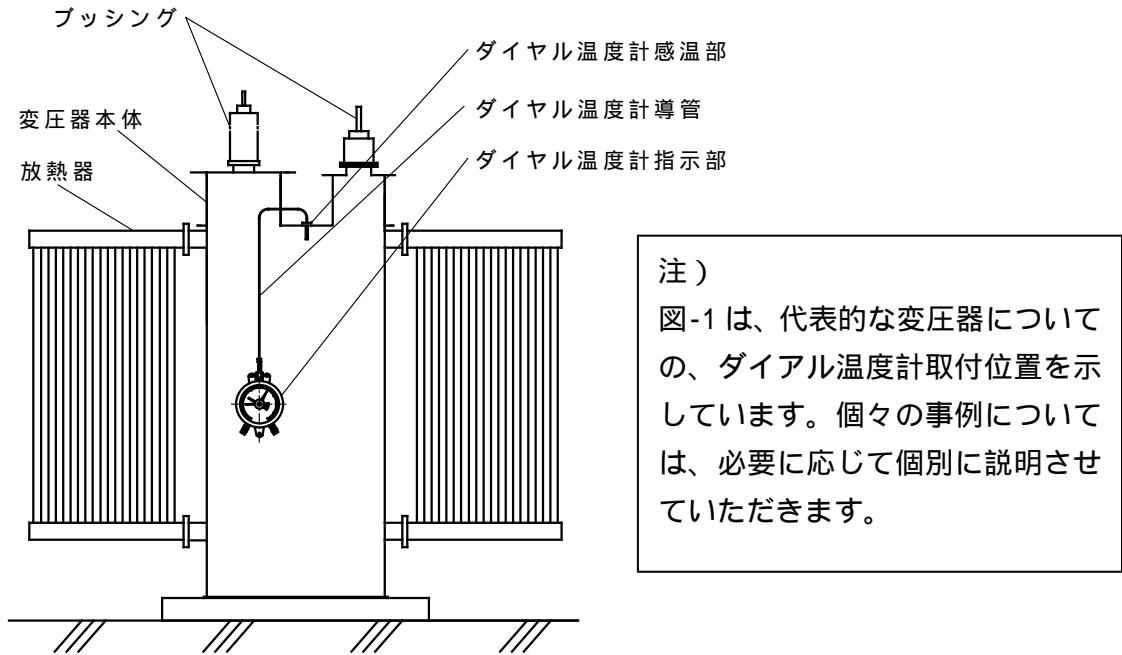
図-1 変圧器 ダイアル温度計 取付位置
