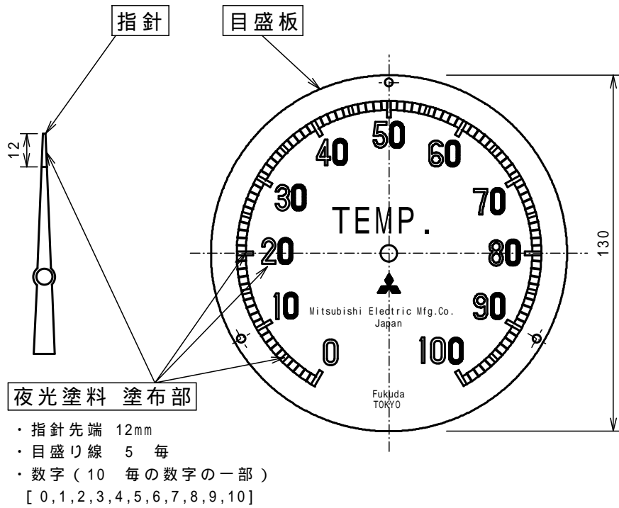
図-3 夜光塗料 塗布位置
