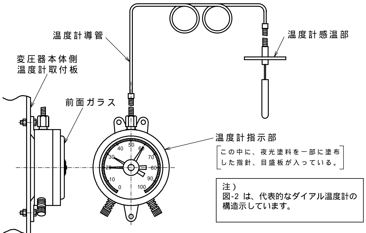
図-2 変圧器 ダイアル温度計 構造図
