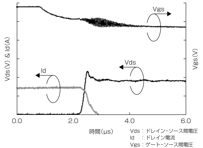
図6. ゲート発振の波形
