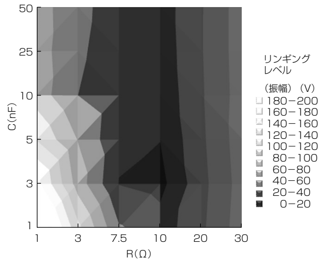
図5. リンギングレベルとRCスナバ定数の相関
