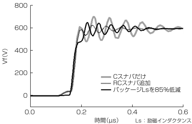
図4. 各条件でのリンギング波形
