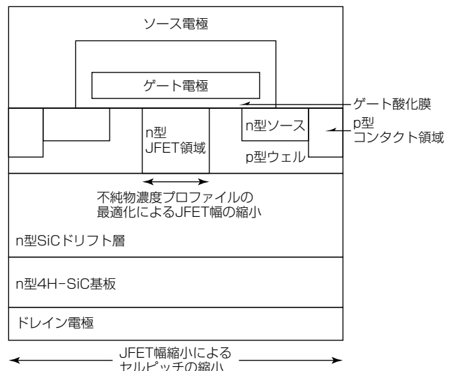
図2. SiC-MOSFETの断面図
