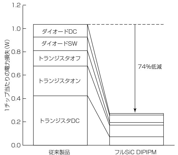
図6. 電力損失比較
