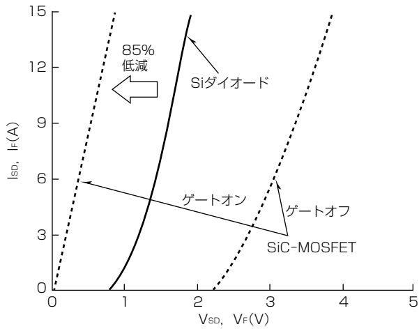
図4. 逆導通特性
