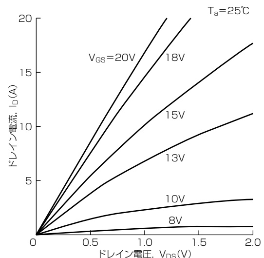
図3. SiC-MOSFETのドレイン電圧-電流特性
