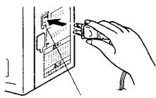
自立運転出力コンセント 100V、最大15A以下
